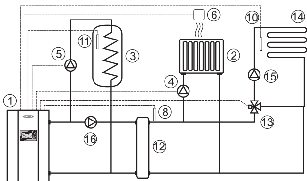
Рис.9 Упрощенная схема подключения котла с гидроразделителем, контуром ГВС и теплого пола.
