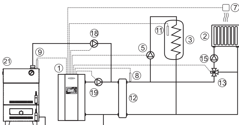
Рис.8 Упрощенная схема подключения котла в режиме вспомогательного с гидроразделителем.
