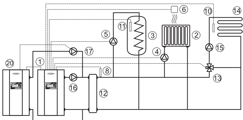
Рис.9 Упрощенная схема подключения котла с гидроразделителем, контуром ГВС и теплого пола.
