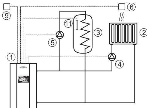
Рис.6 Упрощенная схема подключения котла с контуром ГВС.
