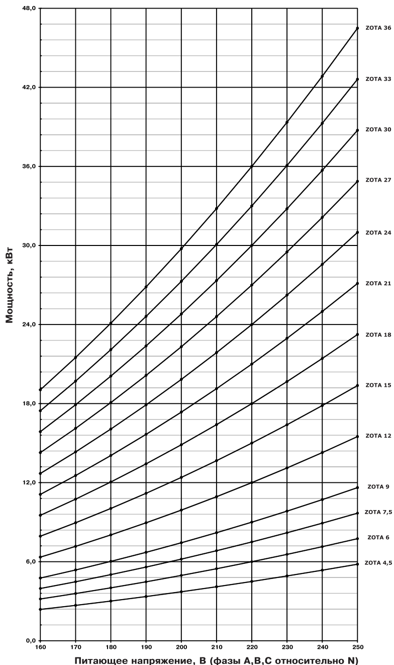
Рис.12 График изменения мощности котла в зависимости от питающего напряжения
