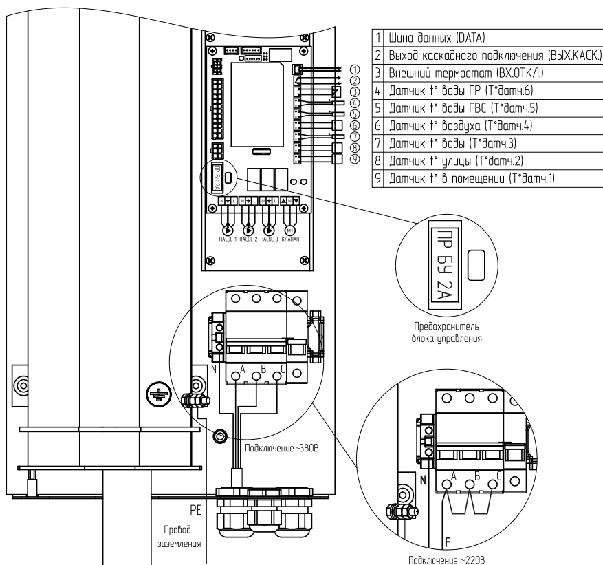
Рис. 3 Схема подключения котла
