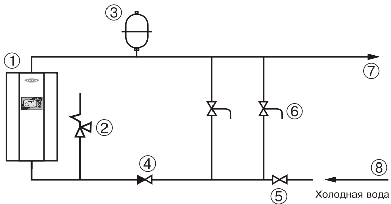
Рис. 11 Упрощенная схема подключения в качестве котла с проточным режимом работы.
