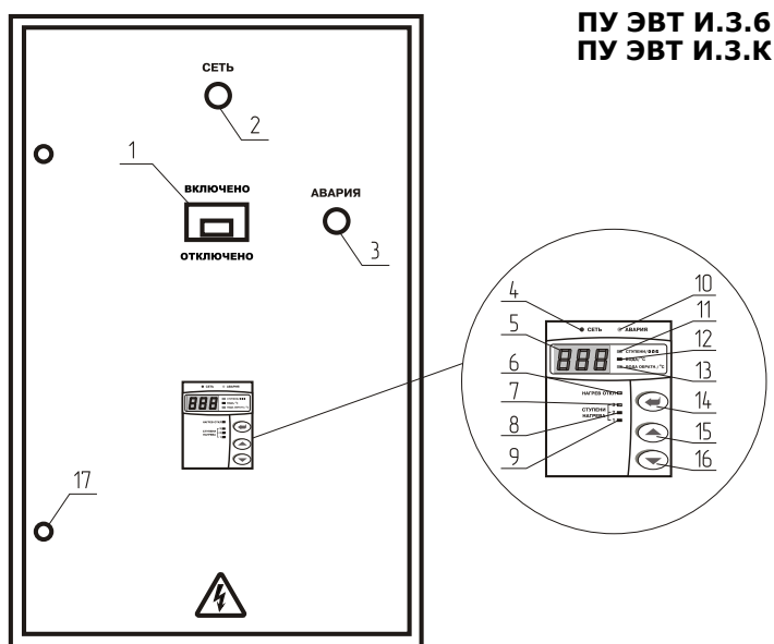
Рис.1 Расположение органов управления панелей правления
